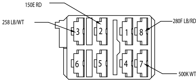
10.27 CARGO LIGHT SWITCH (ETP) 999-16716-001
