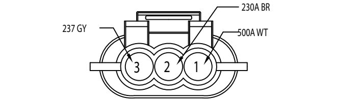
9.2/R RIGHT STOP/TAIL 282087-1
