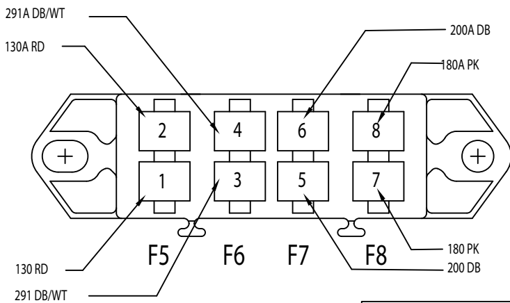
11.12 FUSE PANEL #2 (ETP) 12004943
