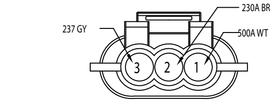
9.2/R RIGHT STOP/TAIL 282087-1
