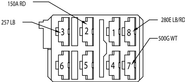
10.7 HEATED MIR SW (ETP) 999-16716-001
