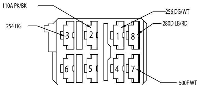
10.8 AUX FAN SWITCH (ETP) 999-16716-001
