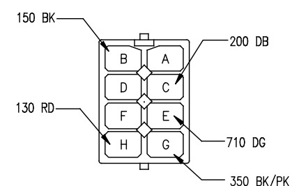
C116 INST-3 F2US-14370-A
