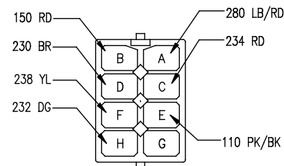
C114 INST-2 F2US-13A718-A
