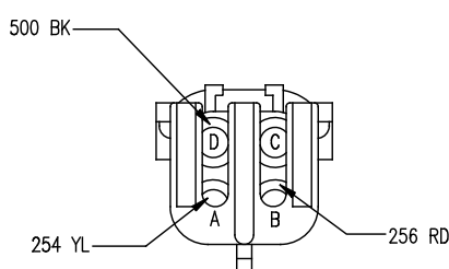
C340 AUX. HTR(SCS) 12015024
