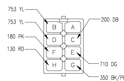
C116 INST-3 F2US-14370-A
