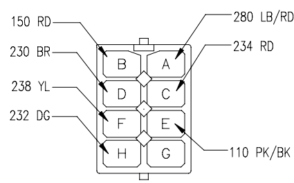
C114 INST-2 F2US-13A718-A
