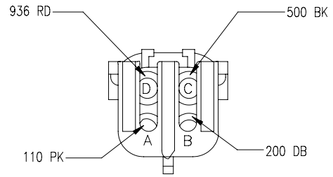
C340 AUX. HTR(SCS) 12015024
